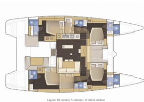
Lagoon 52 versione B (cabinato) - 10 cabine versione
